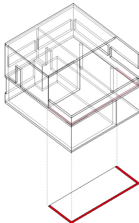
Konstruktions-Grundfläche (KGFc)
