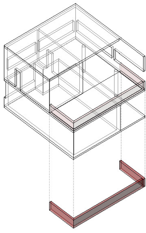
Konstruktions-Rauminhalt (KRlb)
