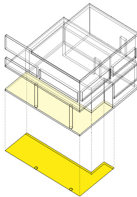
Brutto-Grundfläche (BGFb)
