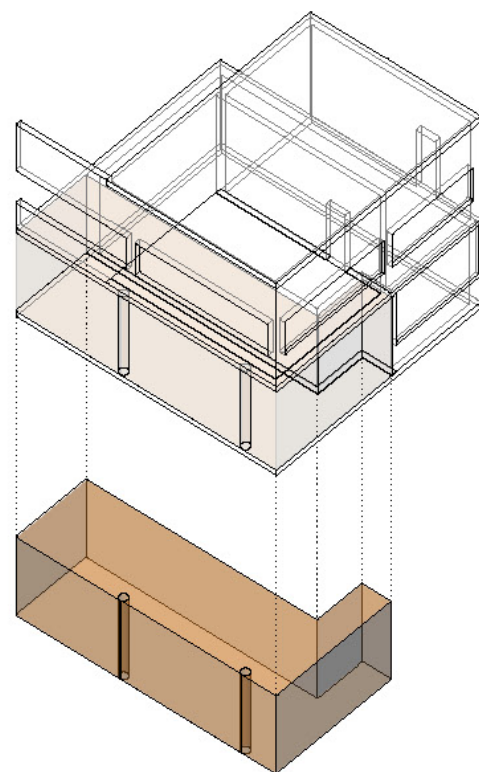
Netto-Rauminhalt (NRlb)
