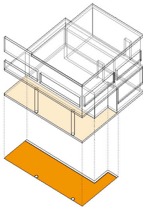
Netto-Grundfläche (NGFb)
