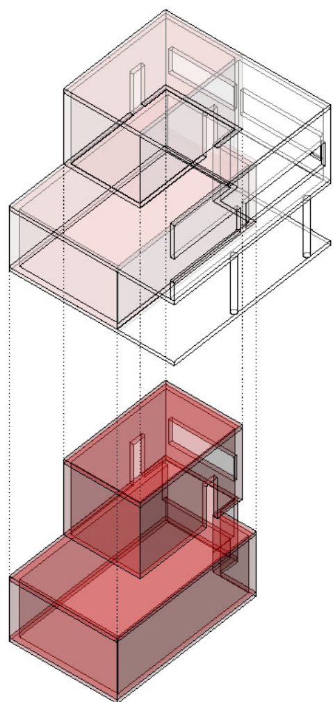
Konstruktions-Rauminhalt (KRlb)
